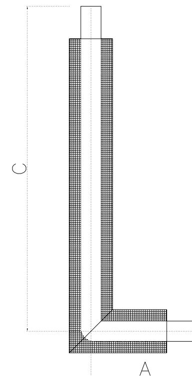
RISER BEND
